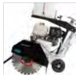
Центр тяжести расположен над осью вращения диска
