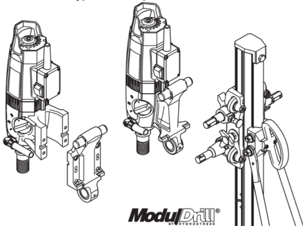
Подсоединение бурильной каретки
