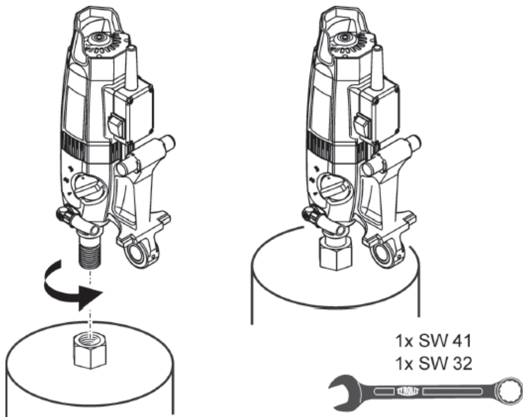
Подсоединение режущего инструмента
